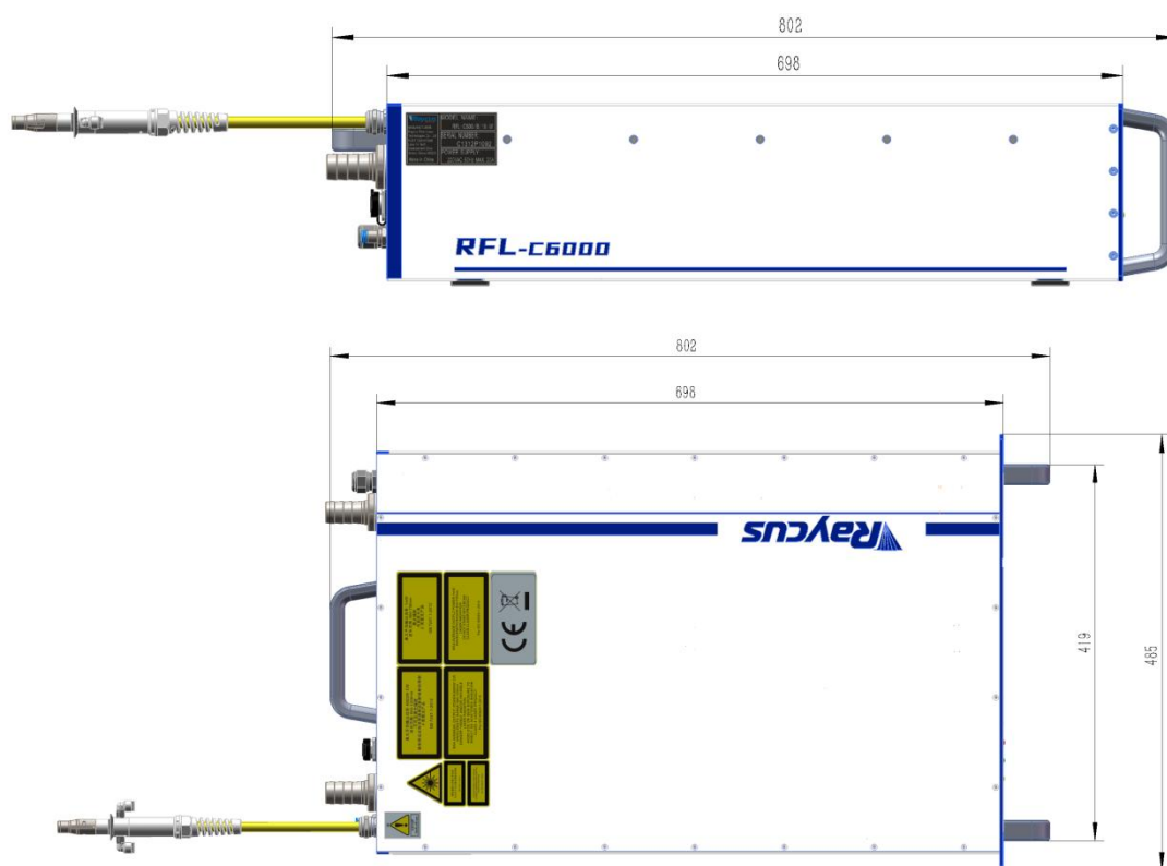
图 2 (b)俯视图、侧视图(单位: mm)
